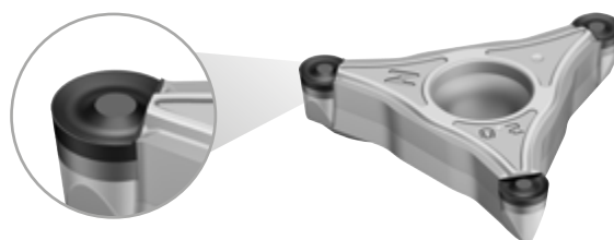
WL25-RCGT..FSM3
