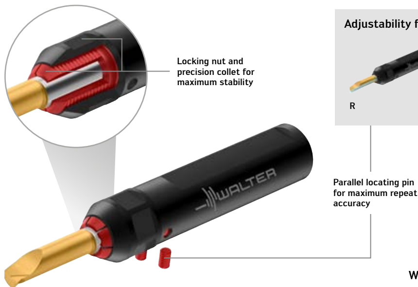
Fig.: WB07-T7225-098R20 WSM23X W4291-A16-WB07
