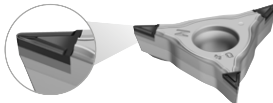
WL25-VCGT..FSM3
